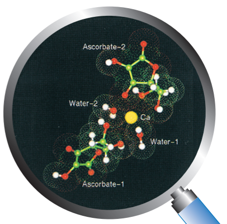
アスコルビン酸カルシウムの立体構造 C 12 H 14 CaO 12 · 2H 2 O 分子量 426.35 武田薬品-分子化学研究室提供(Acta Cryst.B30.2705(1974)より)
