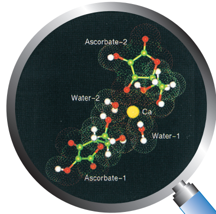
アスコルビン酸カルシウムの立体構造 C_{12}H_{14}CaO_{12} \cdot 2H_2O 分子量 426.35 武田薬品-分子化学研究室提供 (Acta Cryst. B30, 2705 (1974)より)
